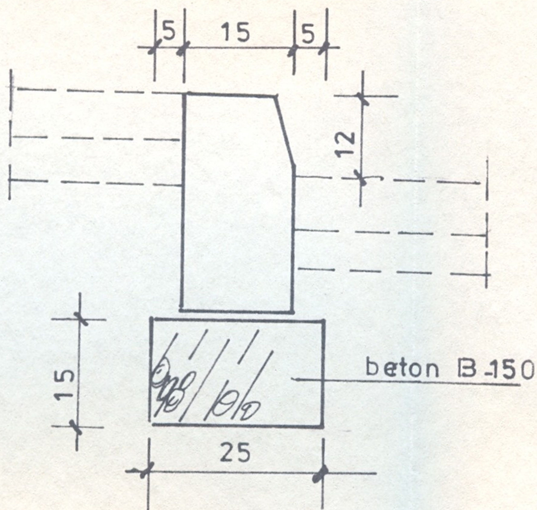
szczegół: „A” 1:10
